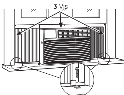
2 ferrures de verrouillage de cadre
