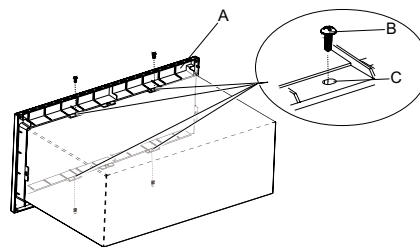
A. Marco del kit de molduras B. Tornillo de cabeza redonda para chapa n.º 7-18 x 7/16" (4) C. Orificio para tornillo (4)
