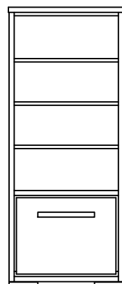
117-02-C Étagère 1 porte (droite) 24" x 19" x 58" (4 tablettes ajustables)
