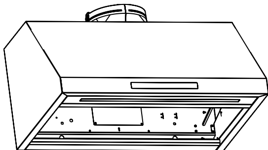
Montage d'un seul moteur
