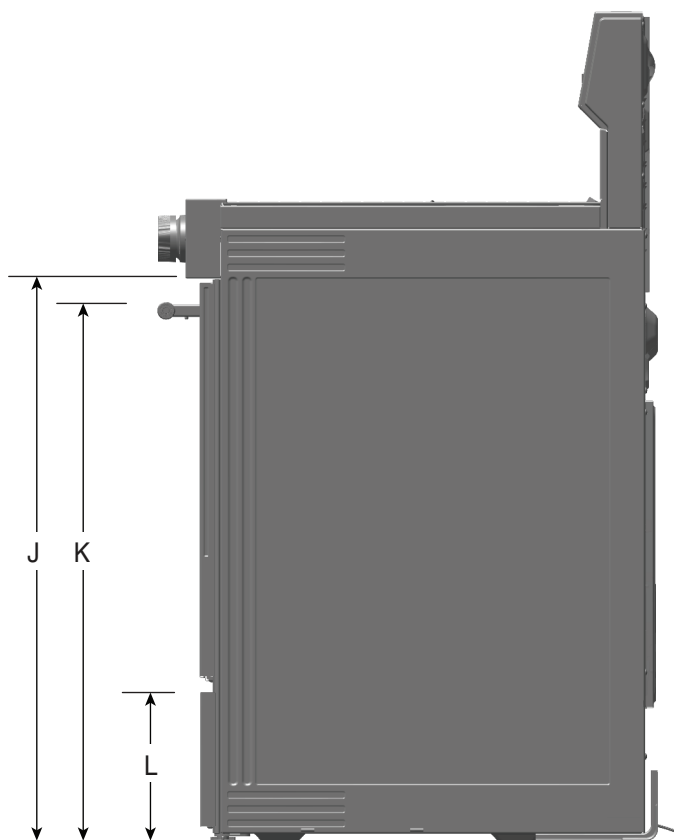
VUE LATÉRALE
