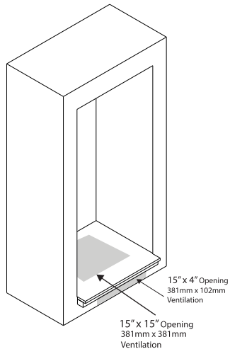
1 Cabinet cutout Découpe de cabinet
