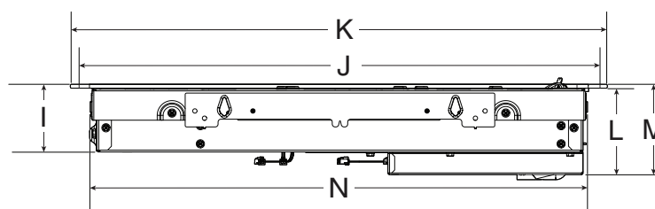
VUE LATÉRALE
