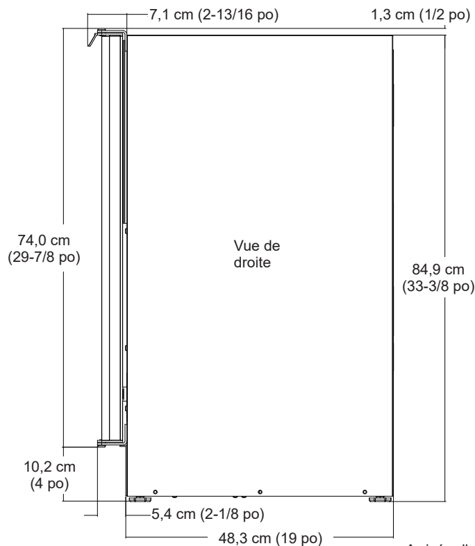
Vue de l'armoire DRC033
