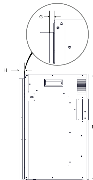
Vue latérale
