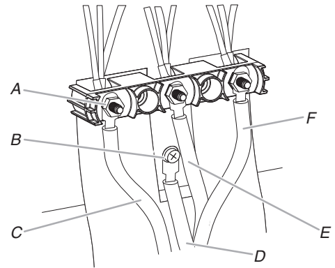
A. Écrou 10-32 à tête hexagonale B. Vis de liaison à la terre C. Ligne 2 (rouge) D. Fil vert (liaison à la terre) E. Fil neutre (centre) F. Ligne 1 (noir)
