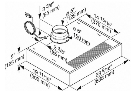
DA 1060, DA 1160, DA 1260 (Installation drawing)
