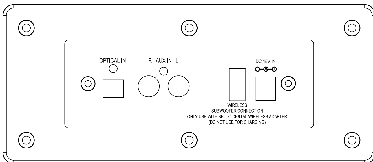
Fig.1 Panneau Arrière
