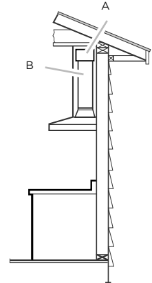
A. Déflecteur B. Conduit rond de 6" (15,2 cm)
