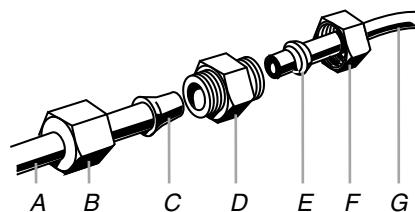
A. Tubería de agua del refrigerador B. Tuerca (provista) C. Bulbo D. Acoplamiento (provisto) E. Fécula (adquirida) F. Tuerca (adquirida) G. Línea de agua de la casa
