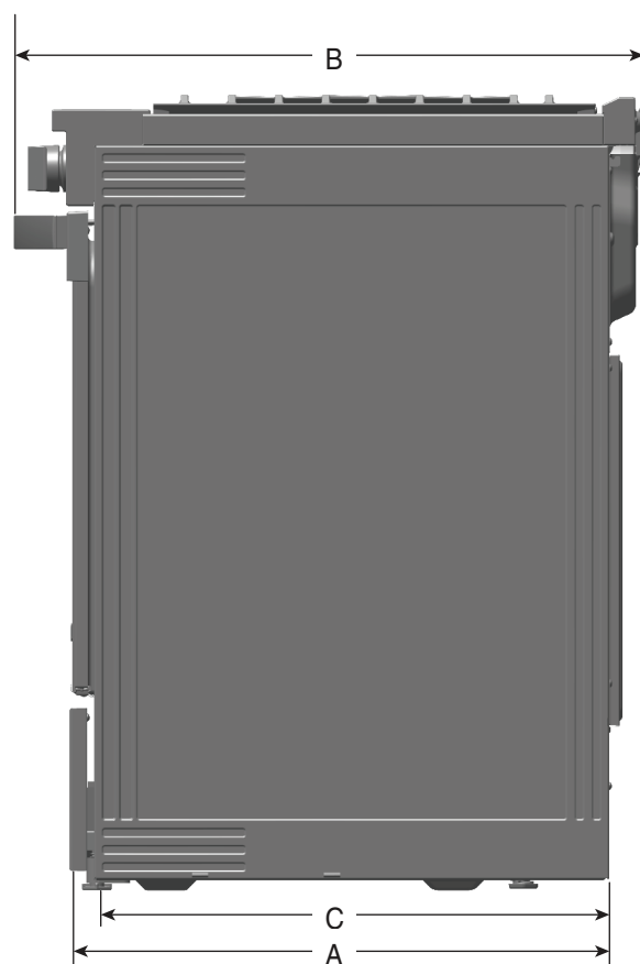
VUE LATÉRALE
