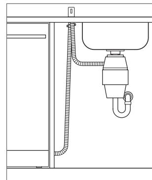
Espace d'air vers élimination
