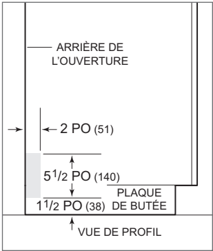
Acheminement électrique
