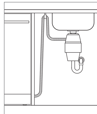
Bucle alto para desechos
