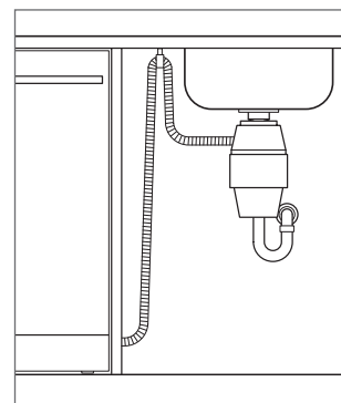
Boucle élevée vers élimination
