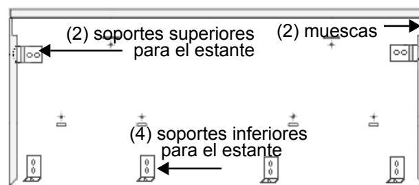
Figura 19: 48 Pulg Dorso de la placa mural
