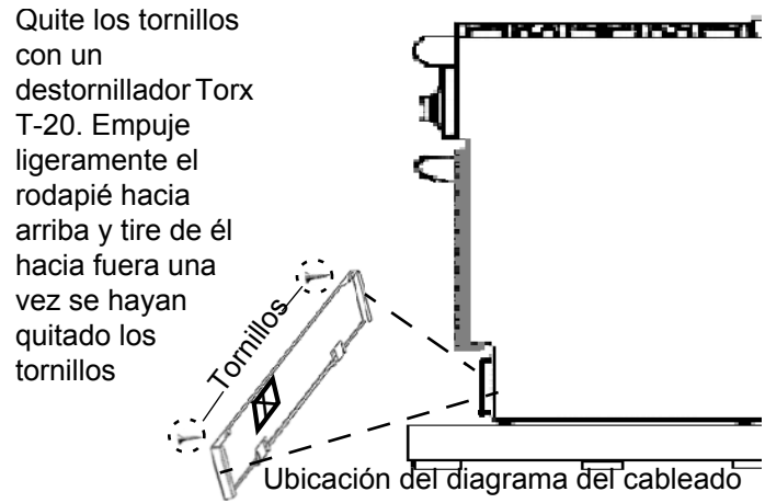
Figura 4: Como quitar el rodapié
