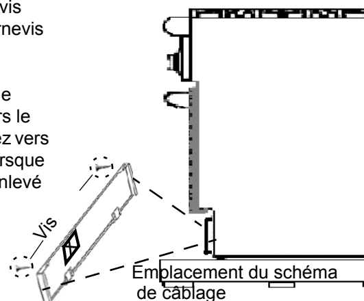
Figure 4 : Retrait du panneau de seuil (plinthe)
