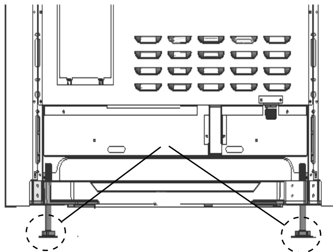
Figura 26: Ubicación de las ruedas
