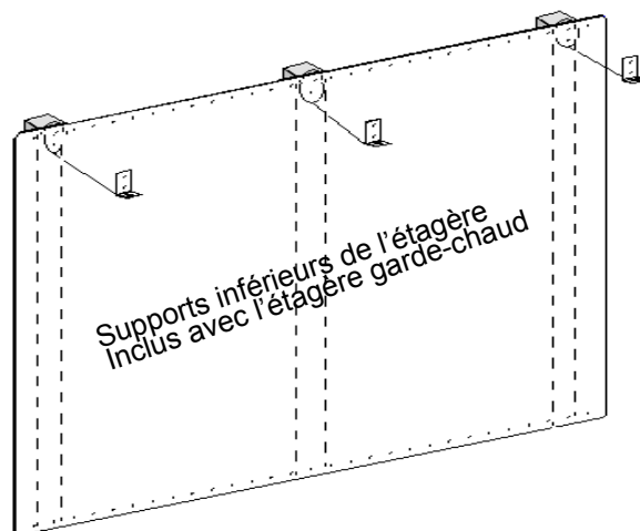
Figure 17 : Dossieret de protection avec étagère garde-chaud
