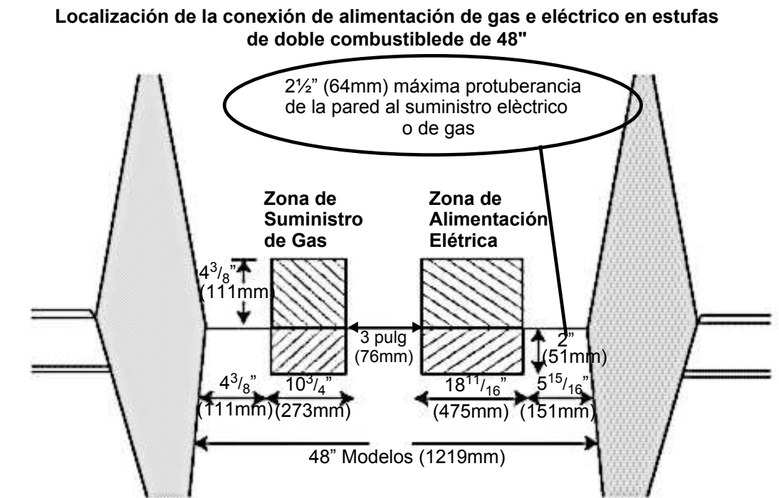
Figura 3a: Suministro eléctrico y de gas para las estufas de doble combustible
