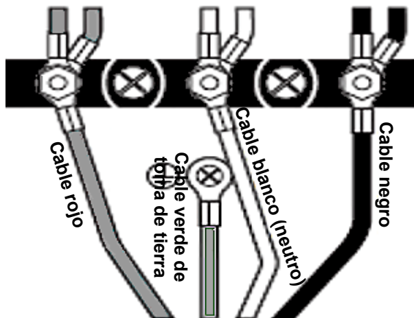
Figura 13: Conexión de cuatro cables
