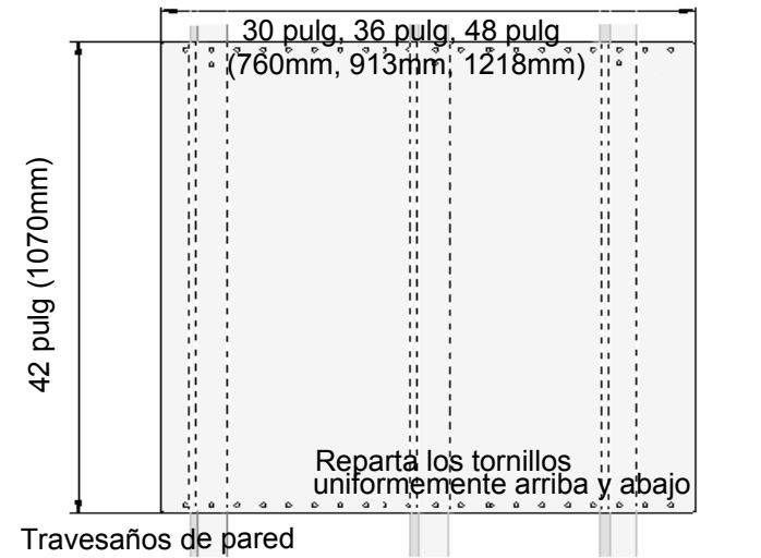
Figura 15: Instalación de la consola trasera
