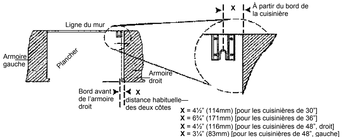
Figure 8 : Mise en place de la patte antibasculer (vue du haut)
