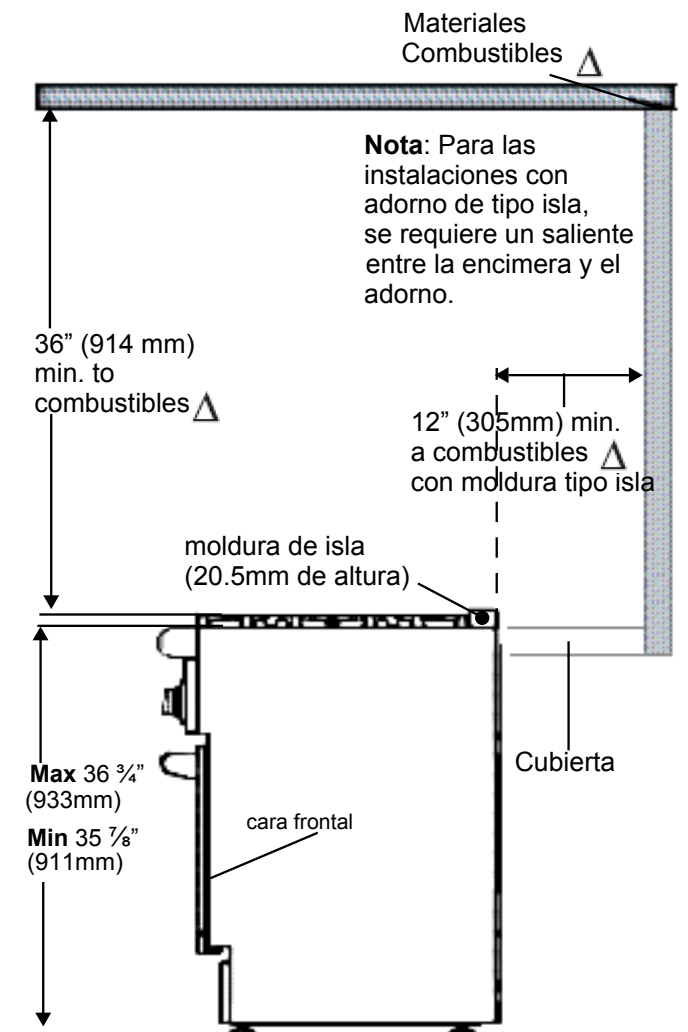
Instalación con "moldura de isla al ras"
