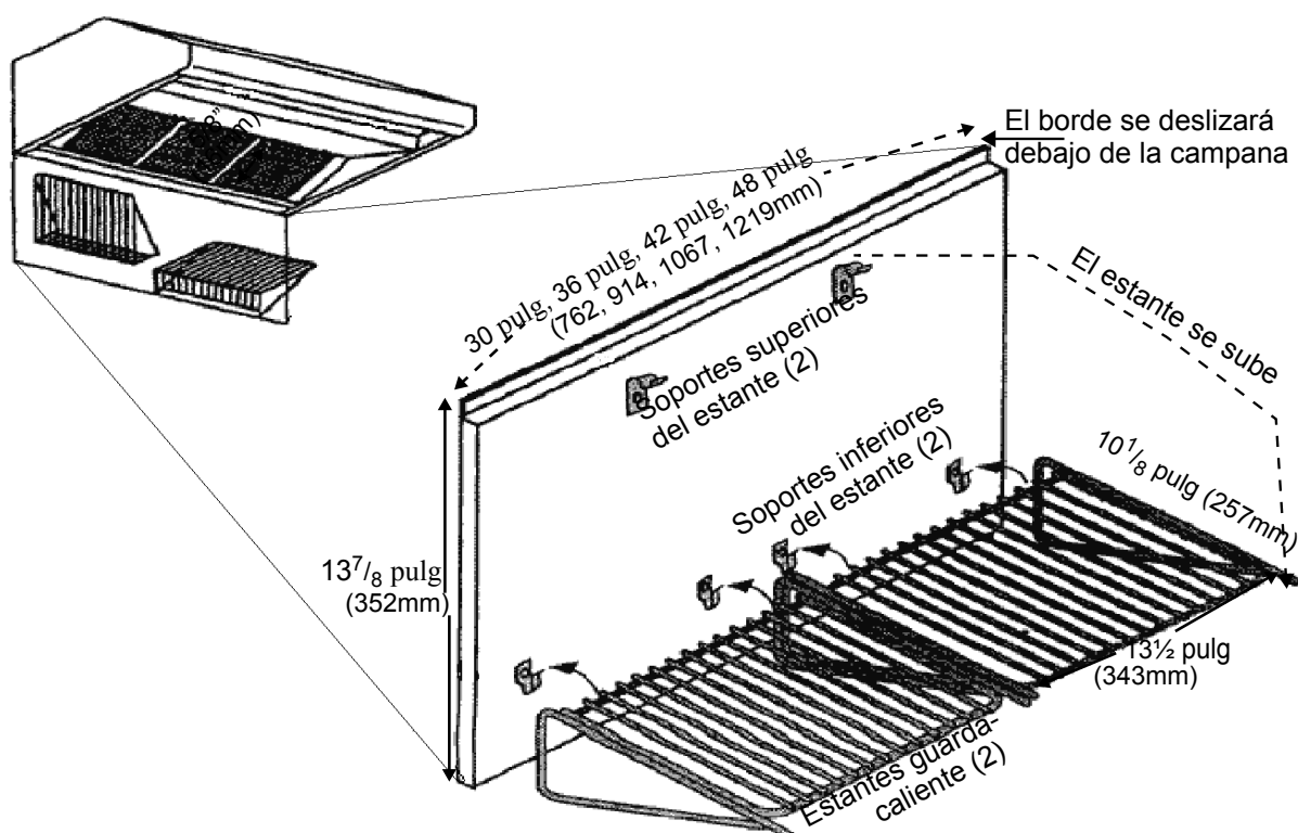
Figura 18: Estante guarda-caliente
