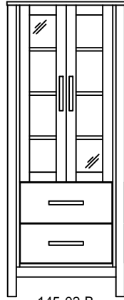
145-02-B Étagère 2 portes vitrées, 2 tiroirs 24" x 19" x 60" (3 tablettes ajustables)
