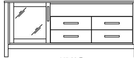
145-09-E Meuble télé 64", 1 porte vitrée, 2 tiroirs 64" x 19" x 27" (1 tablette ajustable)
