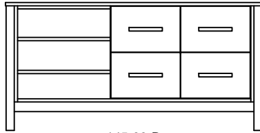
145-09-D Meuble télé 54", 2 tiroirs 54" x 19" x 27" (2 tablettes ajustables)
