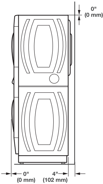
Distances de dégagement arrière/sur le dessus
