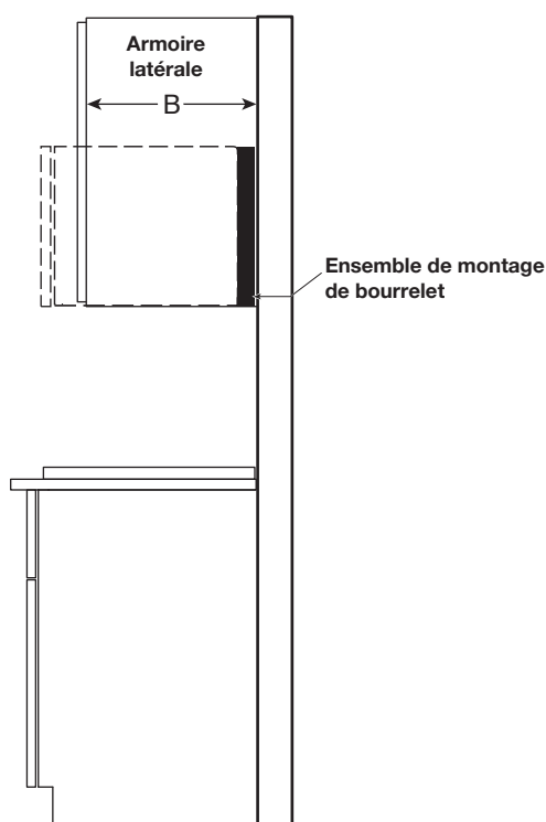
VUE LATÉRALE
