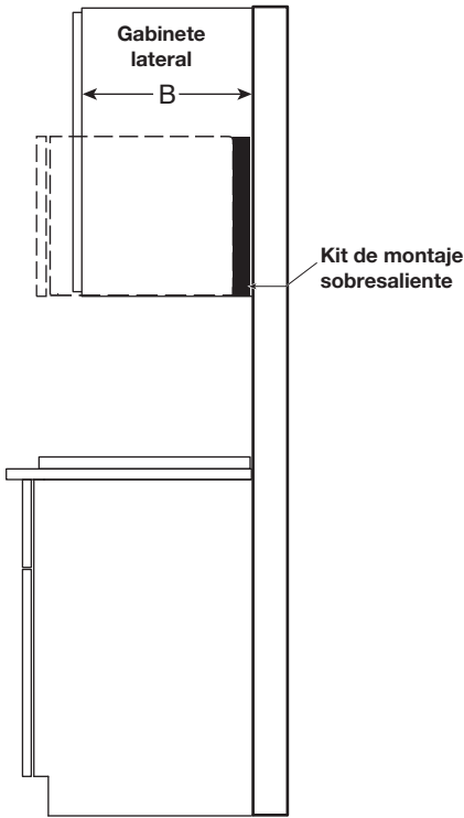
VISTA LATERAL
