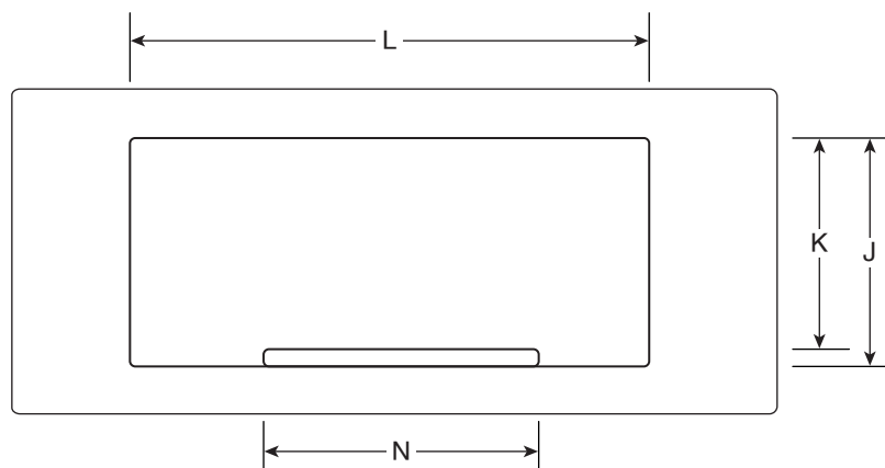
VUE AVANT INTÉRIEURE DE LA CAVITÉ
