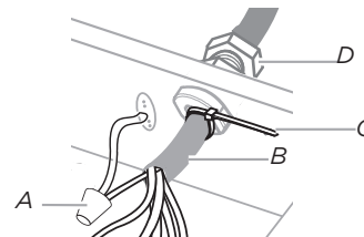
A. Cables de tierra B. Conector de 9-6 cables C. Cincho D. Alivadores de tensión
