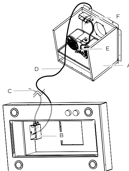
A. Kit de soprador externo B. Caixa de terminais do exaustor C. Conduíte de fiação da fonte de alimentação D. Conduíte de fiação do soprador externo (não incluído) E. Caixa de terminais do soprador externo F. Motor Externo Cabo de tomada eléctrica
