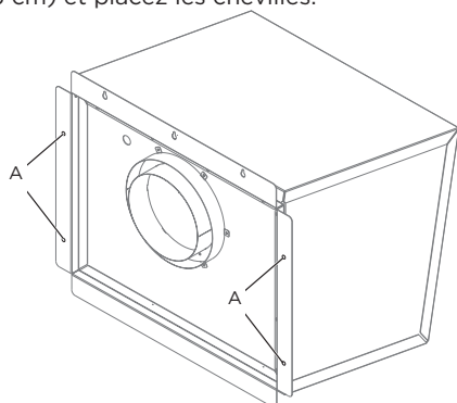
A. Trous de montage
