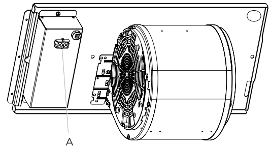
A. Conexión eléctrica
