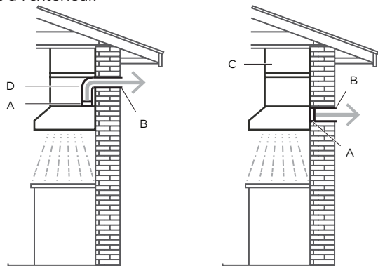
A. Transition B. Conduit rond
