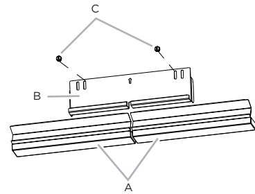
A. Plateau d'égouttement B. Support du plateau d'égouttement C. Vis du support du plateau d'égouttement (2)
