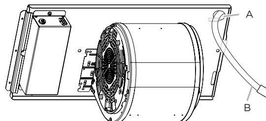
A. Trou de la plaque de montage du moteur B. Câbles d'alimentation et connecteur
