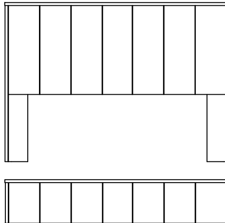
250-39, -54, -60, -78 Lit complet 62" x 44"
