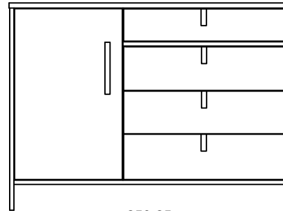
250-25 Commode 4 tiroirs, 1 porte 54" x 19" x 40"
