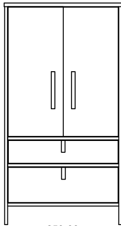
250-06 Chiffonnier 2 tiroirs, 2 portes 32" x 19" x 60" (2 tablettes ajustables)
