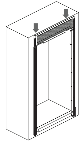
4 Install the top grill Installer la grille supérieure
