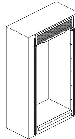
5 Fix the top grill Fixer la grille supérieure
