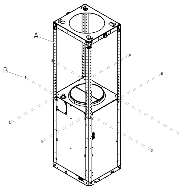
A. Soportes verticales B. 16 - tornillos de 4,2 x 8 mm
