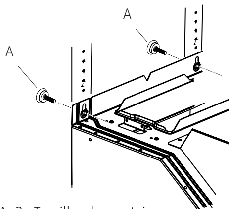
A. 2 - Tornillos de montaje
