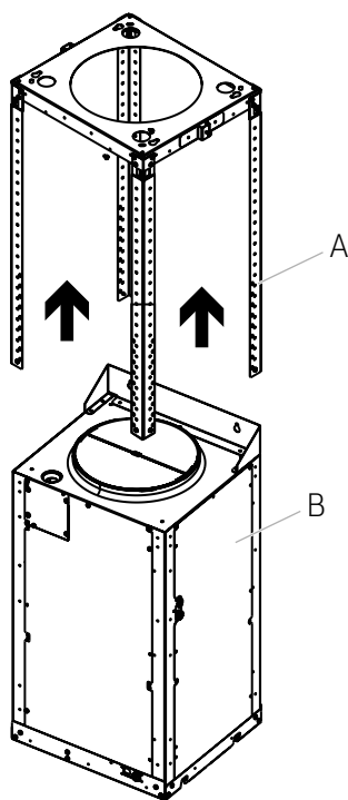
A. Soportes verticales B. Carcasa del soplador
