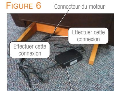
Cordon d'alimentation 120 volts
