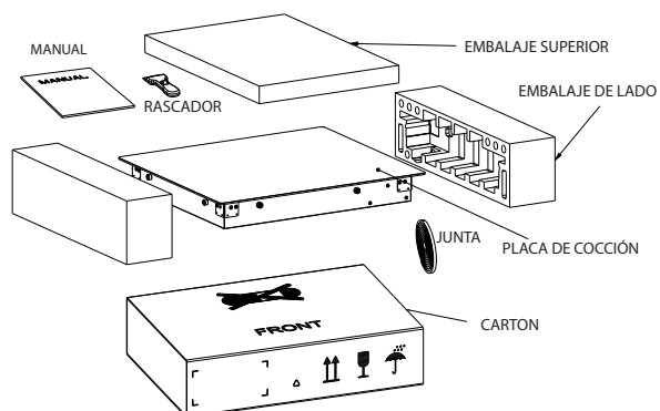
FIGURA 5 - PIEZAS
