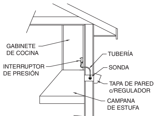
INSTALACIÓN TÍPICA CON VENTILADOR INTERNO Y CONDUCTOS HORIZONTALES CON VENTILACIÓN DE PARED
