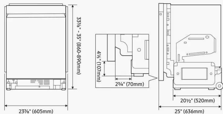
DW80B7070**, DW80B6060**
