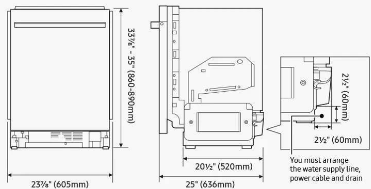
DW80B7071**, DW80B6061**
