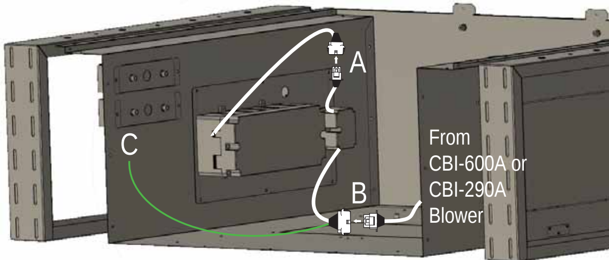
CBI-600A, CBI-290A Wiring
