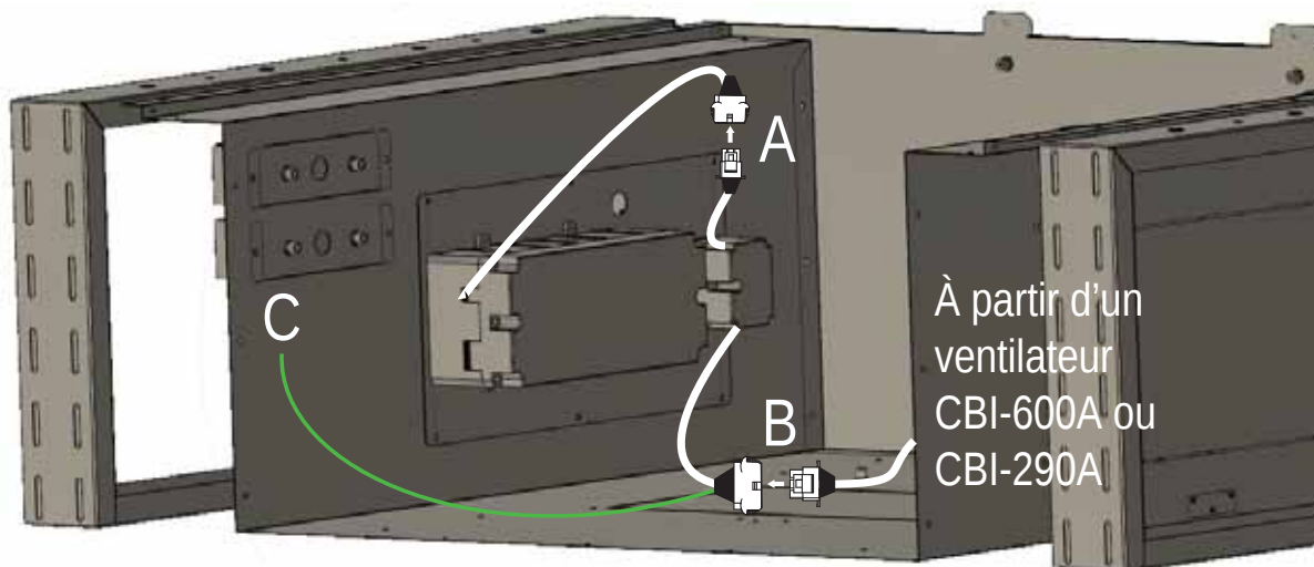
Câblage – CBI-600A, CBI-290A
