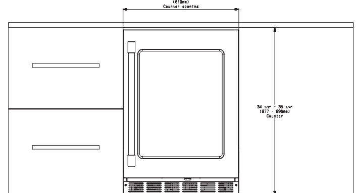
Vue frontale
