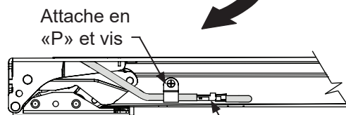
Figure 14b Bas de la porte
