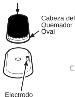
Tapa del Quemador Oval (No Extraíble)
