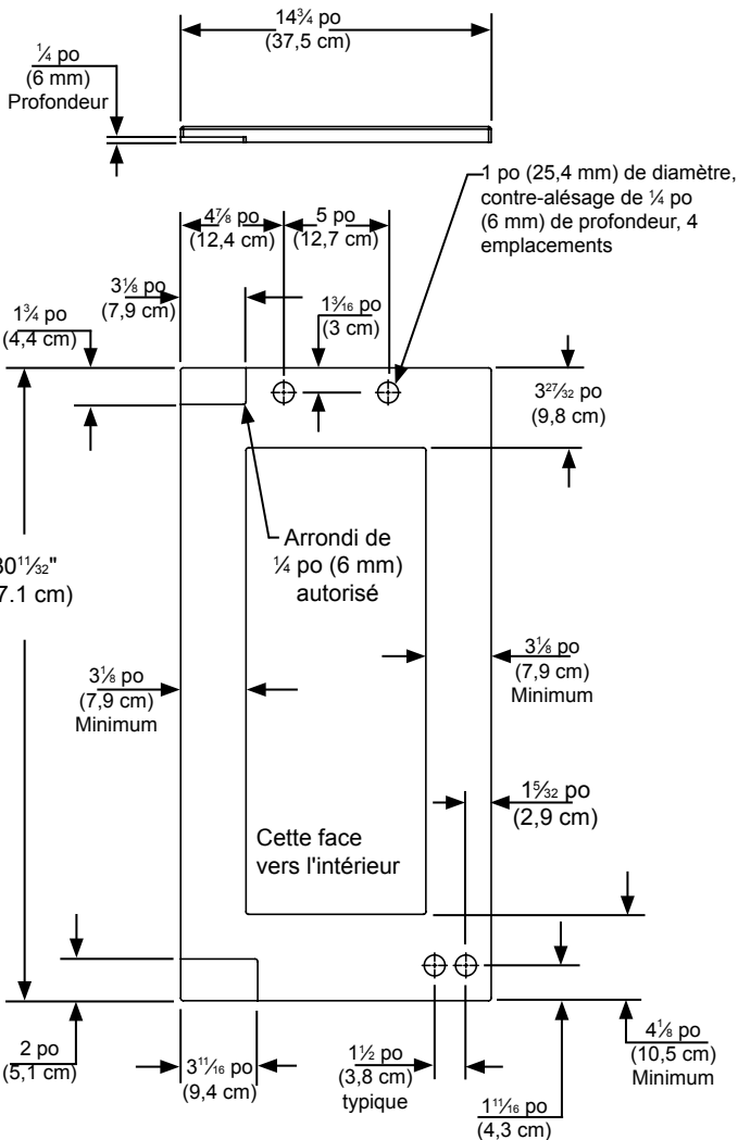
Figure 19 Porte à charnières à droite Appareil de largeur 15 po (38,1 cm)
