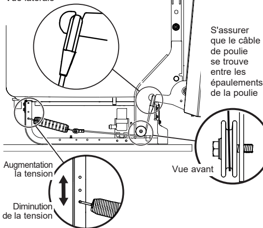
Vue latérale
