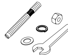
x 1 RP393172-HWKIT Common rail hardware kit complete * Kit de matériel à rampe complet Kit de hardware de carril común completo
