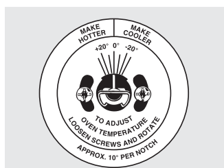
Aguja indicadora (pointer). Vista del reverso de la perilla del termostato del horno.
