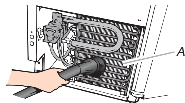
A. Aletas del condensador
