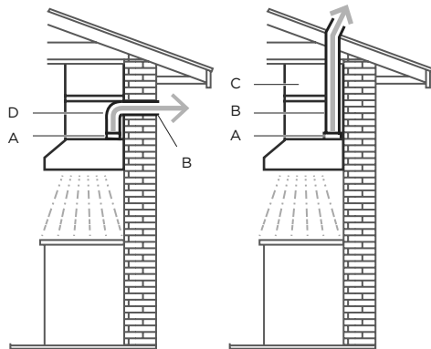
A. Transición rectangular de 3\frac{1}{4}" \times 10" (8.3 x 25.4 cm) B. Ducto de 3\frac{1}{4}" \times 10" (8.3 x 25.4 cm)
