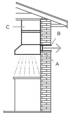
A. Transición rectangular de 3\frac{1}{4}" \times 10" (8.3 x 25.4 cm) B. Ducto de 3\frac{1}{4}" \times 10" (8.3 x 25.4 cm) C. Gabinete
