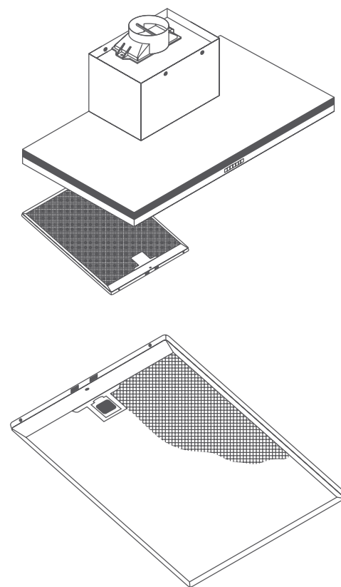
Fig.6 Filtre à graisse
