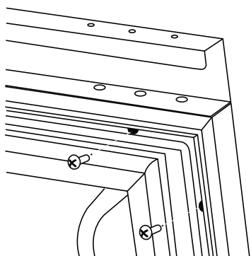
A. Vis B. Joint d'étanchéité
