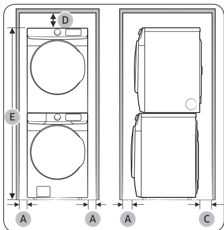
Installation superposée
