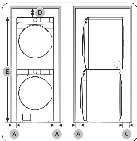
Instalación apilada
