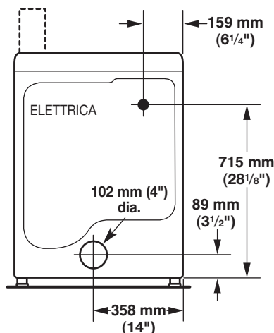
VISTA POSTERIORE
