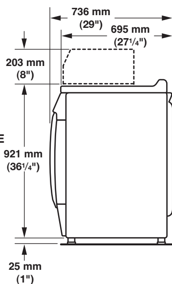
VUE LATÉRALE
