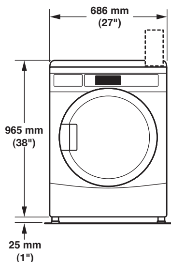
VUE AVANT
