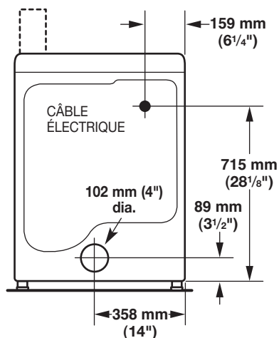
VUE ARRIÈRE
