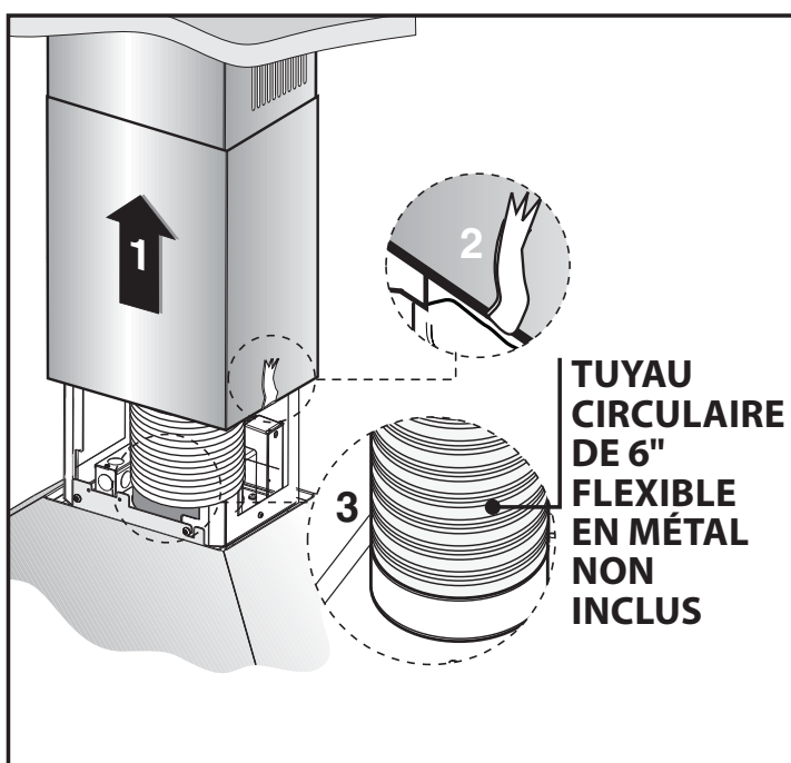
Fig.5: Assembler la cheminée inférieure 1 à celle-ci supérieure et la fixer attentivement en utilisant le ruban adhésif 2 . Fixer le tube flexible ( TUYAU CIRCULAIRE DE 6" FLEXIBLE EN MÉTAL NON INCLUS ) sur la buse sortie de raccordement 3 .
