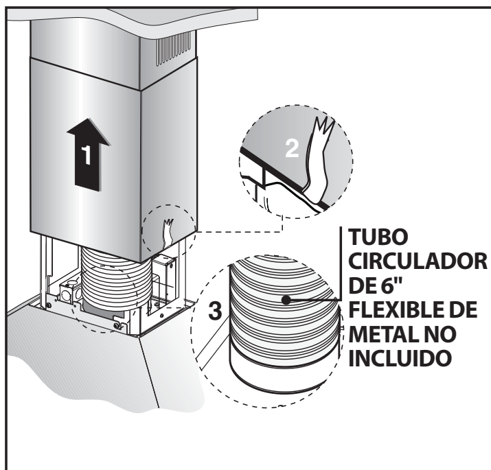
Fig.5: Juntar la chimenea inferior 1 con la superior y fijarla con atención con l'utilización de la cinta adhesiva 2 . Fijar el tubo flexible ( TUBO CIRCULADOR DE 6" FLEXIBLE DE METAL NO INCLUIDO ) sobre la arandela de conexión 3 .
