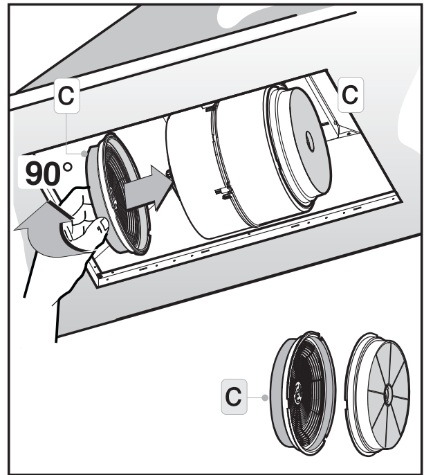
Fig.8: Les filtres C doivent être appliqués au groupe aspirant situé à l'intérieur de la hotte en les plaçant au centre de celui-ci et en les tournant de 90 degrés jusqu'au déclic de blocage.
