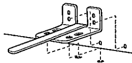
Mínimo Aceptable Nº 1 - Pernos de la Placa de Pared
