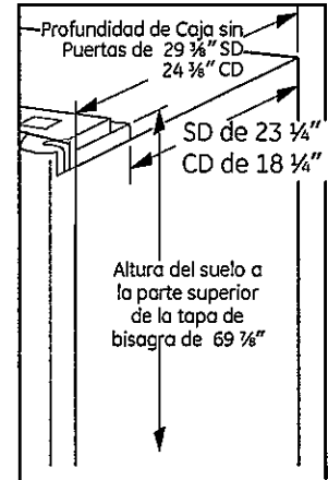
Dimensiones Adicionales
