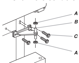
A. Rondelle B. Charnière centrale C. Vis de charnière à tête hexagonale de \frac{5}{16} "
