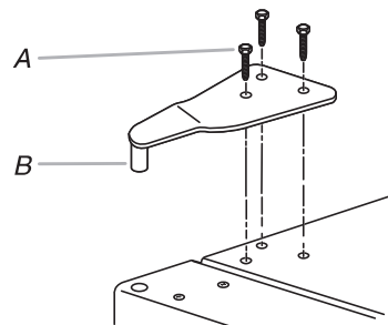
A. Vis de charnière à tête hexagonale de 5/16" B. Axe de charnière supérieure
