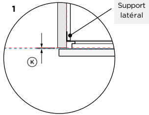
DÉGAGEMENT D'OUVERTURE DES ARMOIRES
