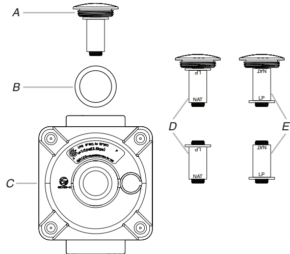
A. Tapa de acceso B. Sello de metal C. Regulador de presión de gas D. Retenedor de resorte en posición NAT E. Retenedor de resorte en posición LP
