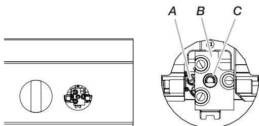
A. Tornillo de ajuste bajo-reducción de fuego lento B. Interrupción de ignición C. Tornillo de ajuste bajo-reducción principal
