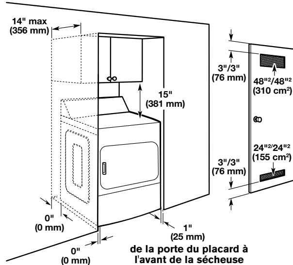
Vue latérale, encastré dans le placard
