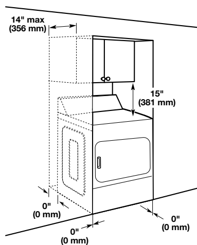
Vue avant, ouverture encastré
