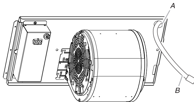
A. Trou de la plaque de montage du moteur
